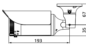
[ LNU3110R / LNU3210R _ Side / Rear ]
