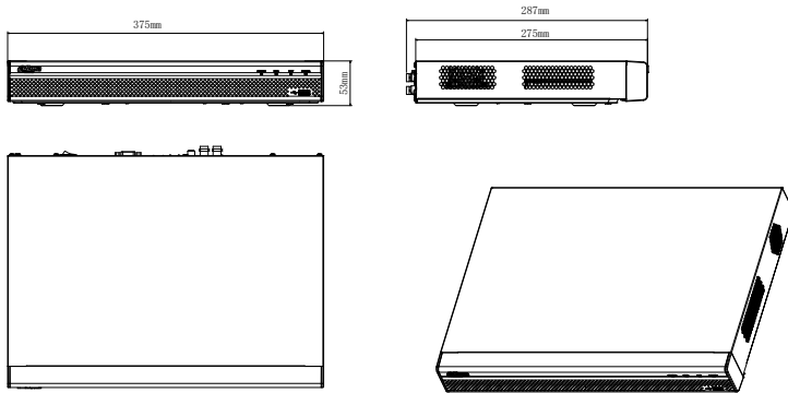
DHI-XVR4216A-S2
