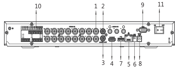
DHI-XVR4216A-S2
