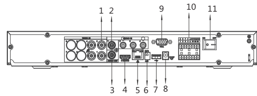
DHI-XVR4204A-S2
