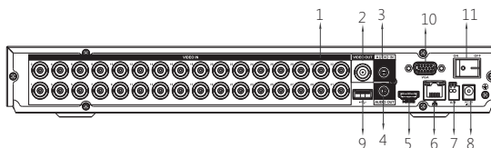
DH-XVR4232AN-X
