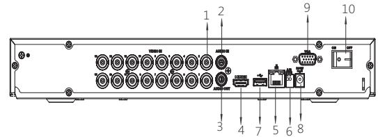
DHI-XVR4216AN-S2
