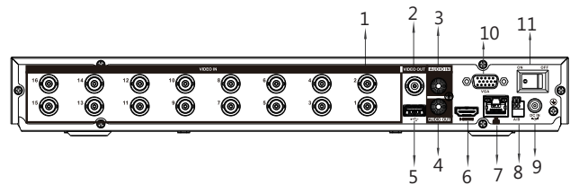
DHI-XVR5216AN-4KL-16P
