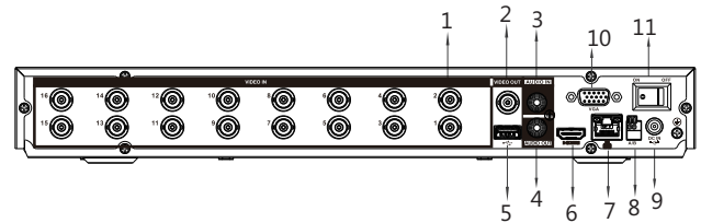
DH-XVR5216AN-4KL-X-16P
