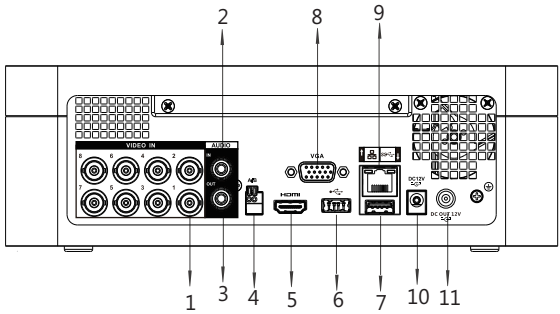
DH-XVR7108E-4KL-B-X
