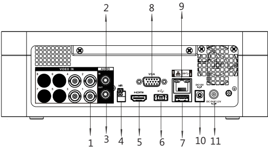
DH-XVR7108E-4KL-B-X
