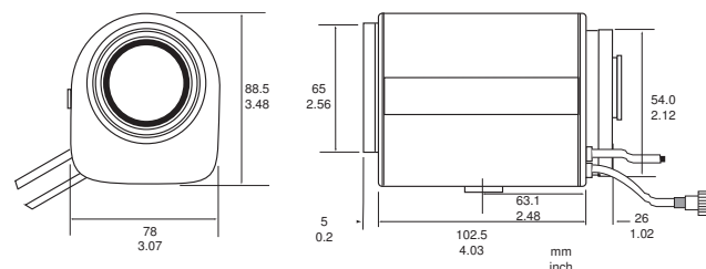
Dimensions LTC 3293 / 20 & LTC 3293 / 30
