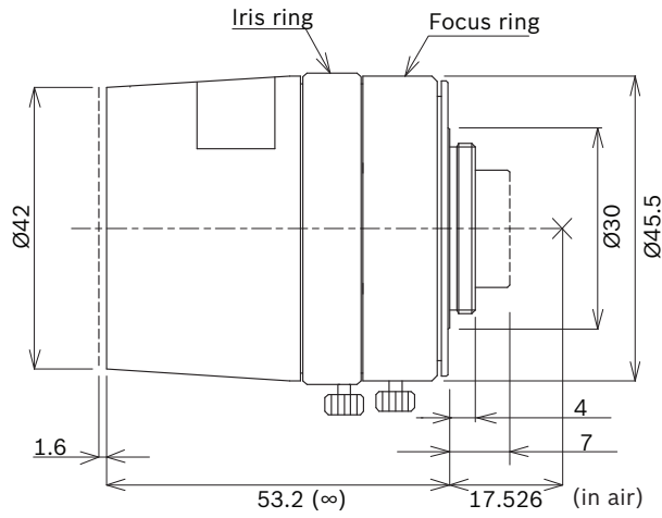
Boyutlar LFF-8012C-D50
