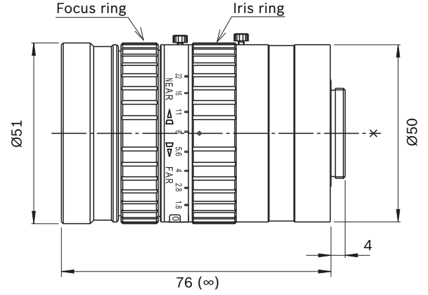
Boyutlar LFF-8012C-D75
